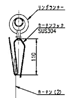
カーテン(2)取付部 カーテンフック詳細
