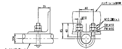
カーテン(2)用レール取付ホルルト 詳細
