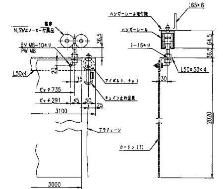
カーテン(1)用レール取付詳細
