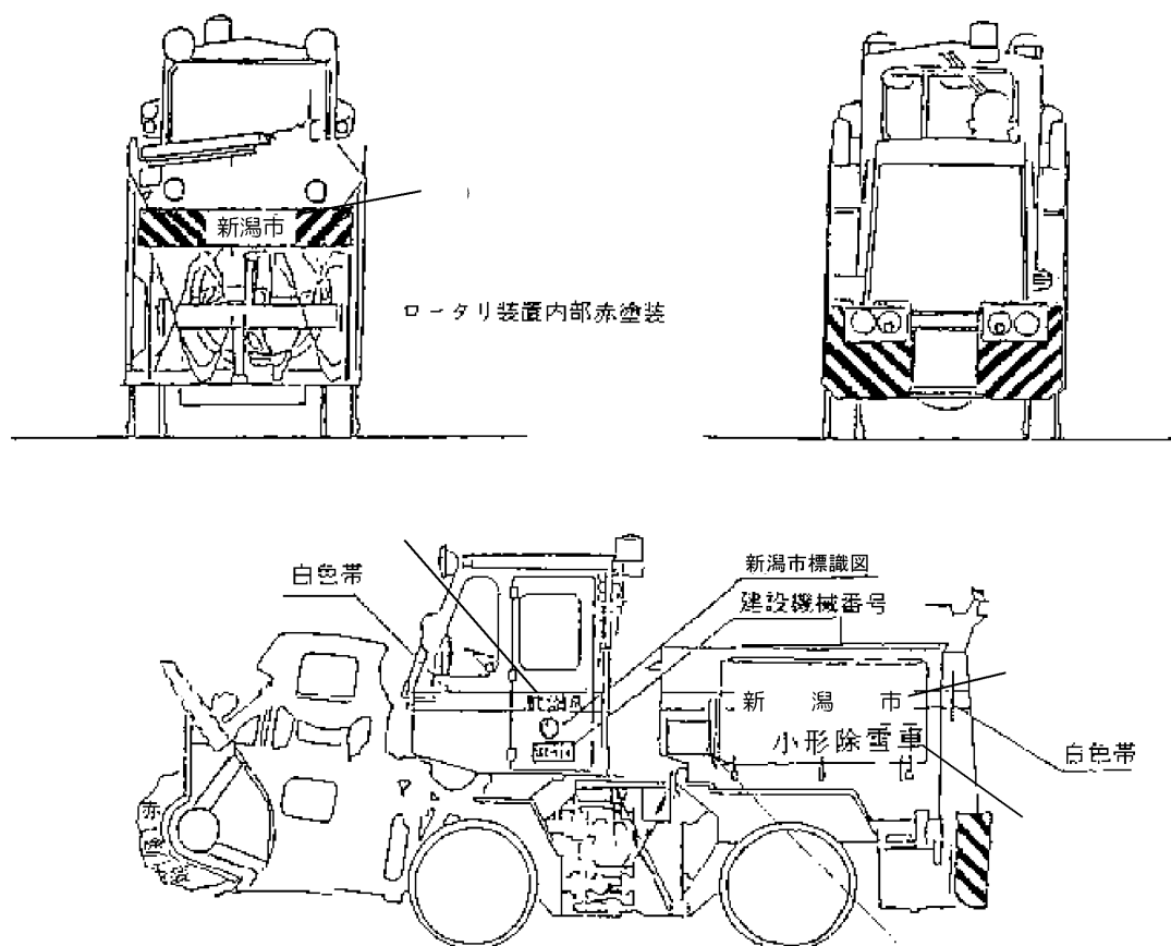
図1 除雪機械表示箇所図
