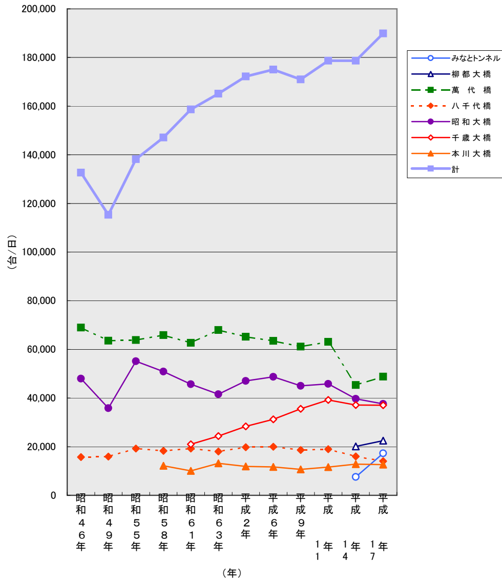
信濃川下流断面
