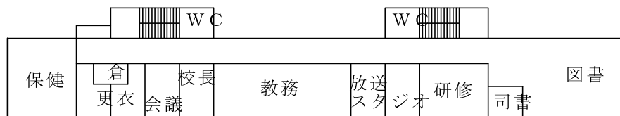
2階平面図
