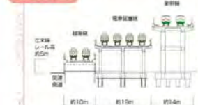
D-D' 断面
