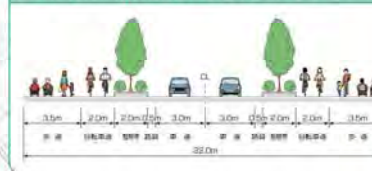
(都)新潟駅西線及び(都)新潟駅東線(車線数:2車線、幅員:22m)
