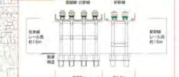
B-B' 断面
