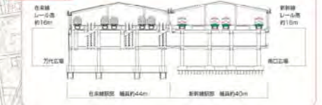
A-A' 断面
