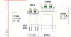
C-C' 断面
