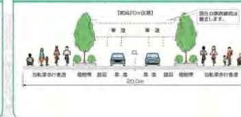
(都)明石紫竹山線(車線数:2車線、幅員:18m及び20m-幅広機直)
