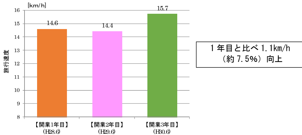
快速便の平均旅行速度（新潟駅前～青山の上下線平均）
