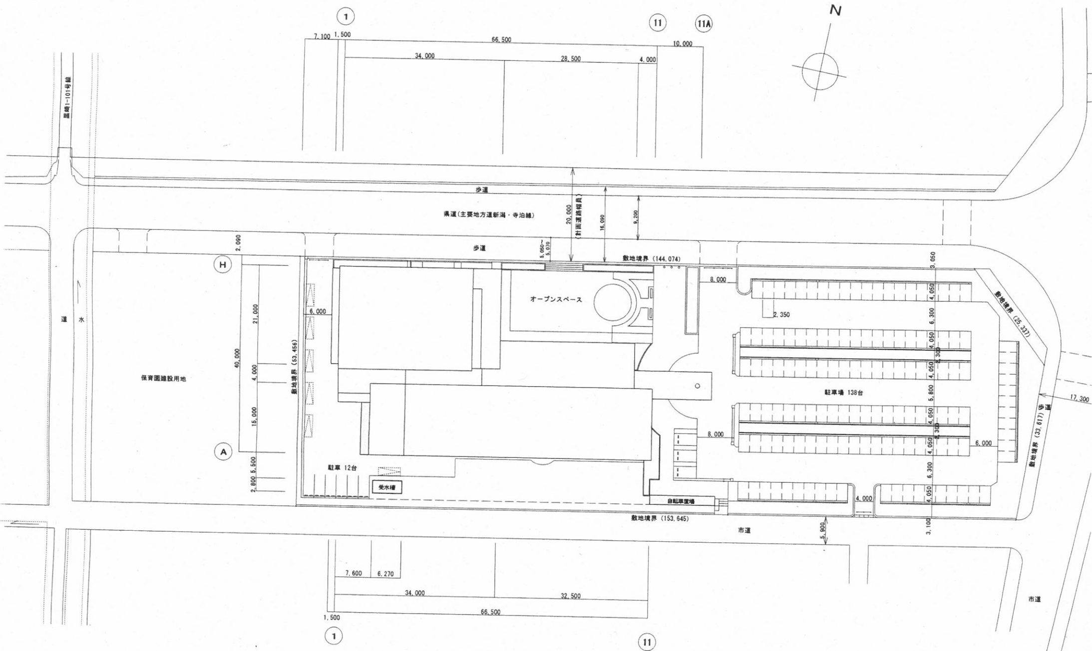
配置図 S=1/400
