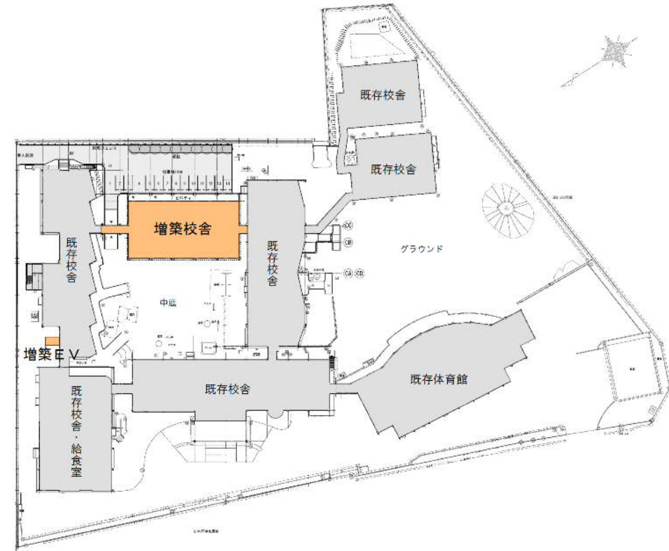
■増築校舎 1階平面図
