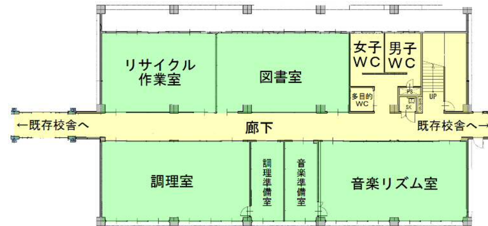
■増築校舎 2階平面図
