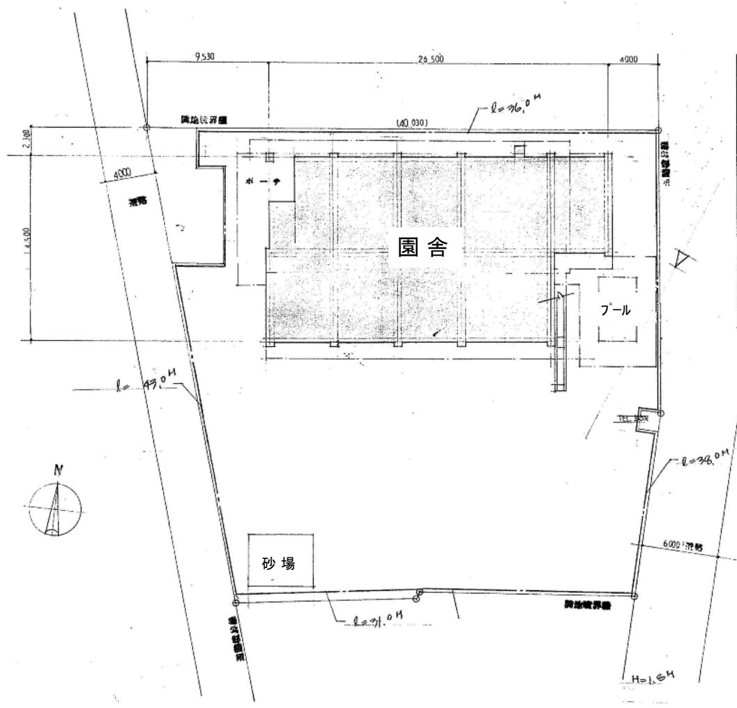
配置図
