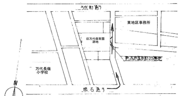
附近見取図
