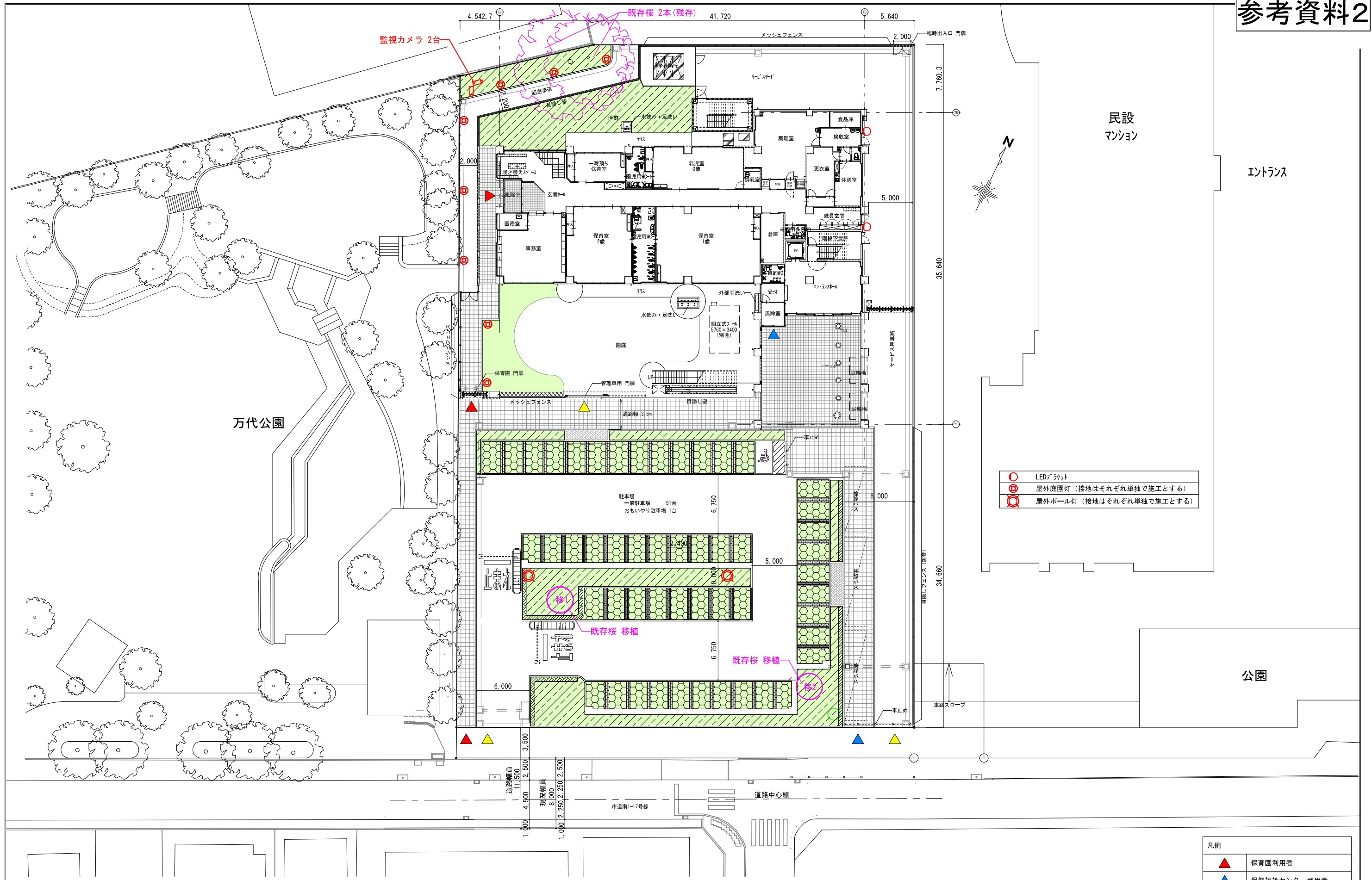
配置図 S=1/100
