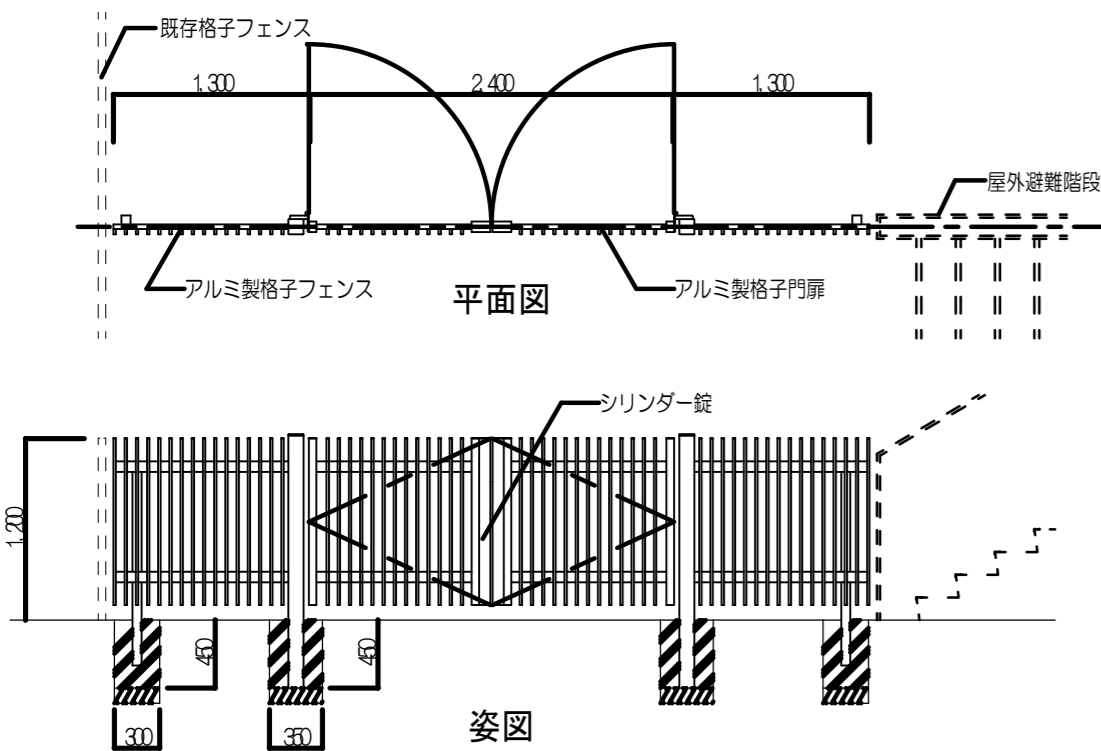
格子フェンス門扉 1:50
