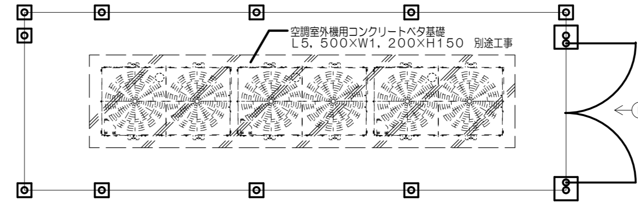
平面図 S=1:50
