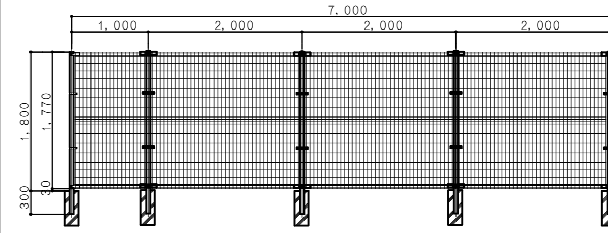
A面展開図 S=1:50
