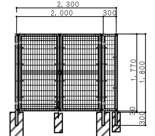
B面展開図 S=1:50
