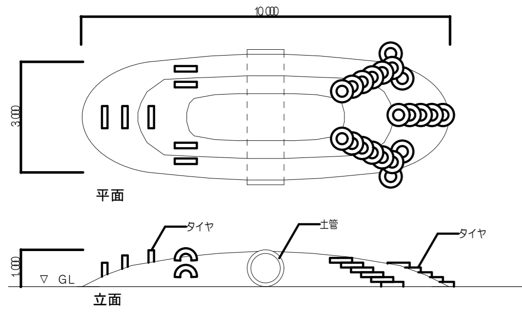
鋼製スベリ台 1:50
